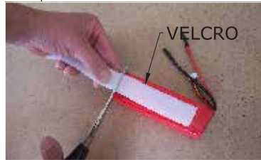
184. K upevnění akumulátorů použijeme např. suchý zip Use dry zipper as battery holder for example.
