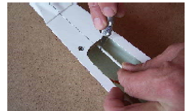
154. Podle polohy serva a délky koncovky + rezerva pro pohyb, zkrátíme vedení táhla Reduce length of the pushrod pipe according to servo position, ending and space for movement.
