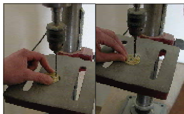
105. V motorové přepážce #1-1 vyvrtáme otvory podle použitého motoru a zahlubíme je Drill holes on motor wicket #1-1 according to applied motor and sink holes.
