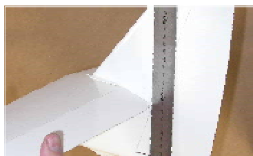
193. ...dolů = 11 - 15mm ... down = 11 - 15 mm.
