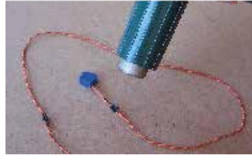
117. ...bužírky smrštíme ... shrink tubes.
